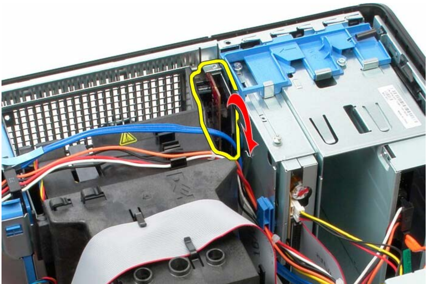
7. Lyft ut I/O-panelen ur platsen.
